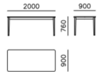
dining table SFA-DT 200
